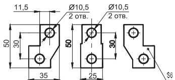
Рисунок Д.2 - Комплект дополнительных расширительных присоединительных выводов
