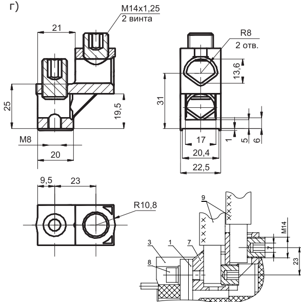
Рисунок Д.1 – Способы присоединения внешних проводников к выключателю:
