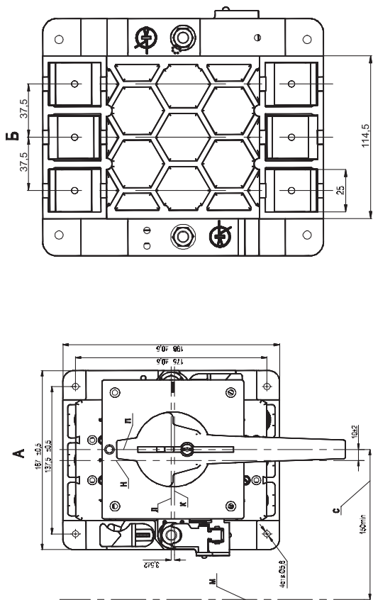
Рисунок Б.7 - Выключатель ВА57-35 выдвигного исполнения с ручным дистанционным приводом Условные обозначения см. рисунок Б.8
