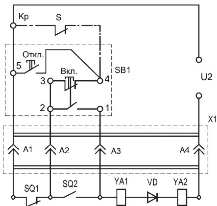
Рисунок Г.9 - Электрическая принципиальная схема привода электромагнитного
