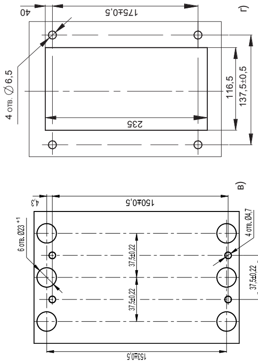
в) стационарного исполнения, заднего присоединения проводников; г) выдвижного исполнения
