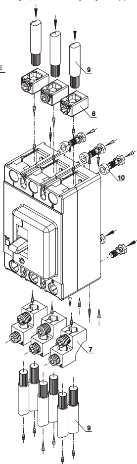
Рисунок Д.2 - Комплект дополнительных расширительных присоединительных выводов
