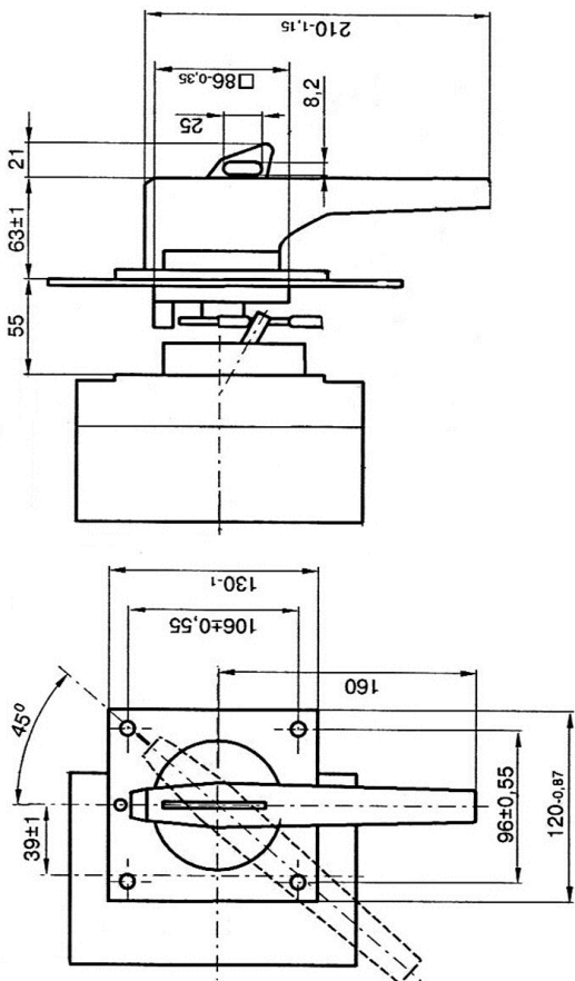
Рисунок Б.5 - Выключатель BA57-35 (BA57Ф35) с ручным дистанционным приводом для оперирования через дверь распределительного устройства
