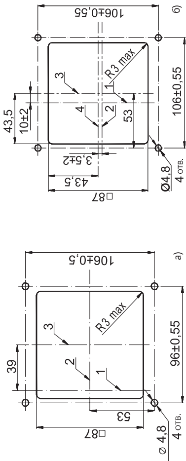
1 - вертикальная ось выключателя; 2 - горизонтальная ось выключателя; 3 - вертикальная ось ручного дистанционного привода; 4 - горизонтальная ось ручного дистанционного привода; а) стационарного исполнения, переднего присоединения проводников; б) выдвижного исполнения
