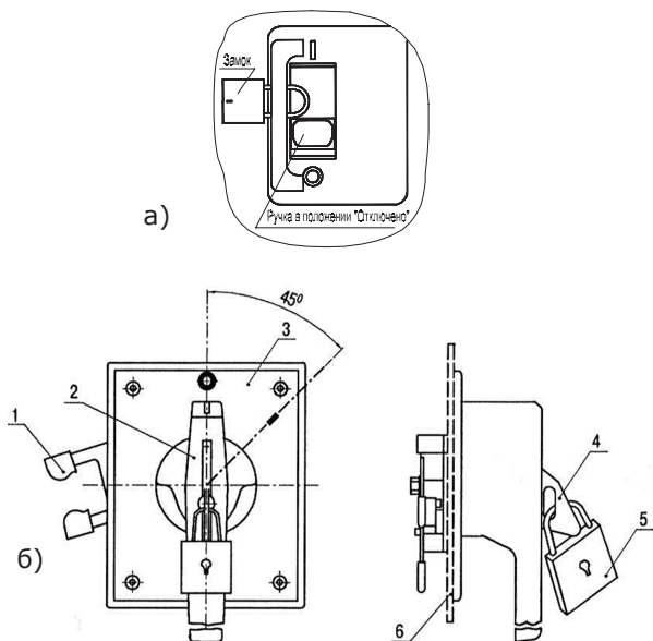
а) выключателей стационарного исполнения, б) выключателей с ручным дистанционным приводом (1 - поводок; 2 - рукоятка; 3 - основание; 4 - пластина; 5 - замок; 6 - дверь распре- делительного устройства)
