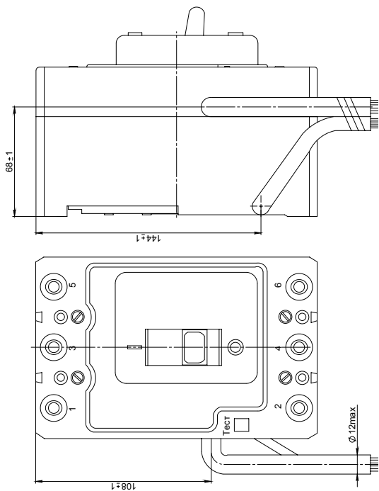
Рисунок Б.9 - Расположение выходящих из выключателя проводов от дополнительных сборочных единиц
