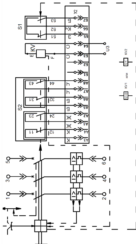
Рисунок Г.8 - Схема электрическая принципиальная выключателей выдвижных исполнения, с нулевым или минимальным расцепителем напряжения, вспомогательными контактами сигнализации автоматического отключения, вспомогательными контактами включения, вспомогательными контактами Примечание: На рисунках Г.3, Г.4, Г.5, Г.6, Г.7, Г.8 положение вспомогательных контактов сигнализации автоматического отключения S1 приведено для выключателя в положении «отключено» после «автоматического» срабатывания
