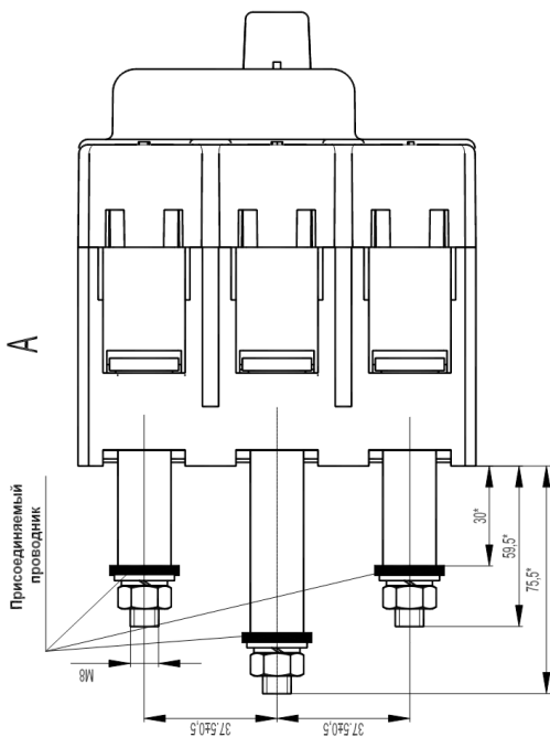
Рисунок Б.2 - Выключатели BA57-35 (BA57Ф35) с зажимами для заднего присоединения
