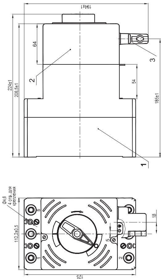
1 - выключатель; 2 - привод электромагнитный; 3 - соединитель типа РП10 Рисунок Б.6 - Выключатель BA57-35 (BA57Ф35) с электромагнитным приводом
